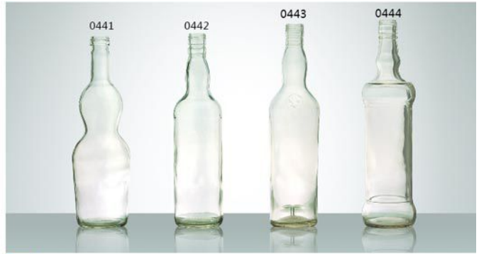
N-0441 SIZE : 288x90mm G : 510g V : 750ml N-0442 SIZE : 290x75mm G : 500g V : 685ml N-0443 SIZE : 305x77mm G : 555g V : 750ml N-0444 SIZE : 310x80mm G : 550g V : 730ml
